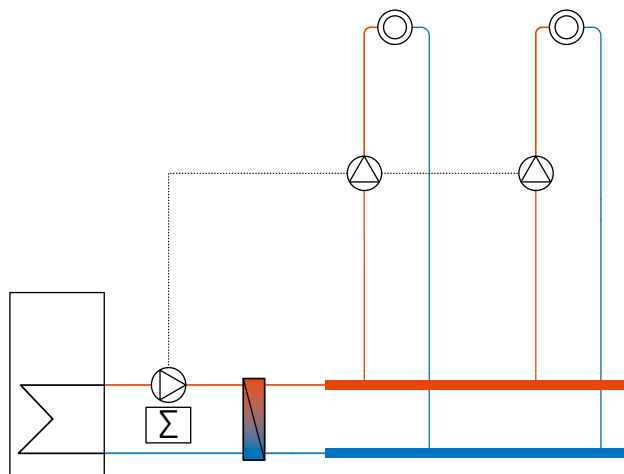
Multi-Flow Adaptation der Zubringerpumpe vor einem Wärmetauscher mit Sekundärpumpen im Strang ohne Mischer
