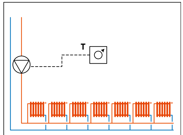
Hallentemperaturregelung bei Verbraucherkreis Heizkörper
