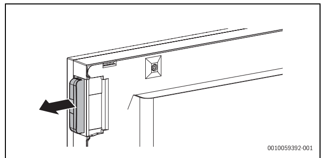
Bild 4 Kommunikationsmodul demontieren
