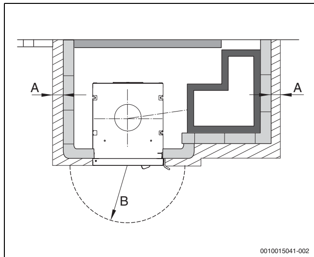
Bild 5 Äußere Mindestabstände
