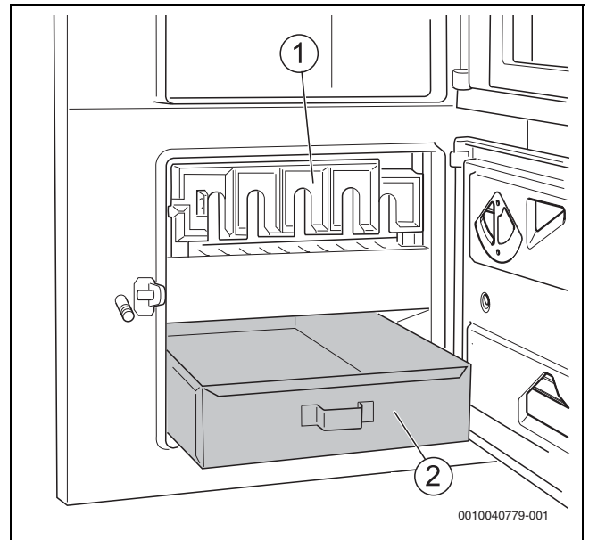
Bild 11 Aschekasten entnehmen
