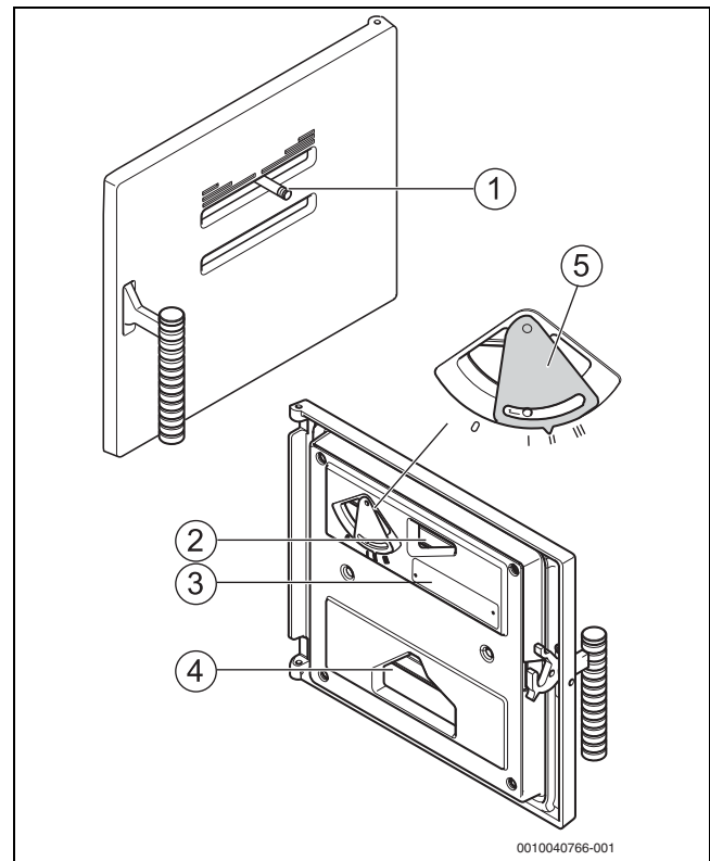
Bild 8 Aschetür
