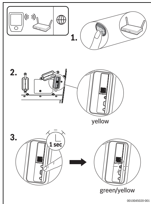
Fig. 188 Racord WPS
