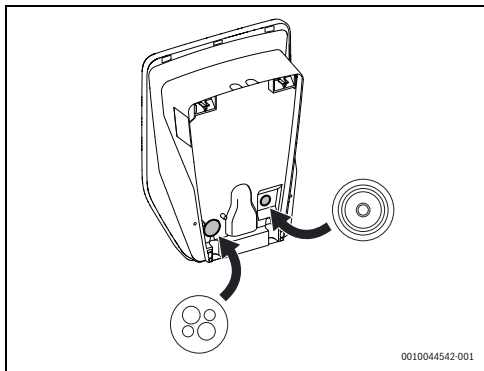
Obr. 203 Inštalácia zátky káblovej priechodky a káblovej priechodky s viacerými otvormi (CLIXX)
