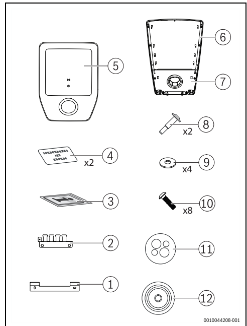
Rys. 145 Zakres elementów
