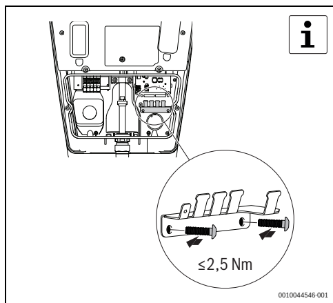
Obr. 207 Inštalácia držiaka kábla
