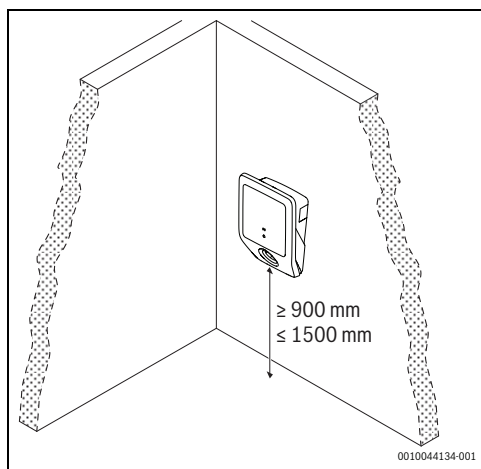
Rys. 149 Minimalne odległości
