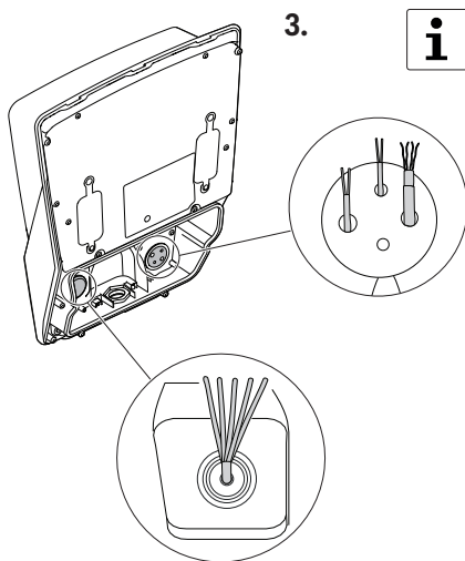
Obr. 36 Montáž na zeď
