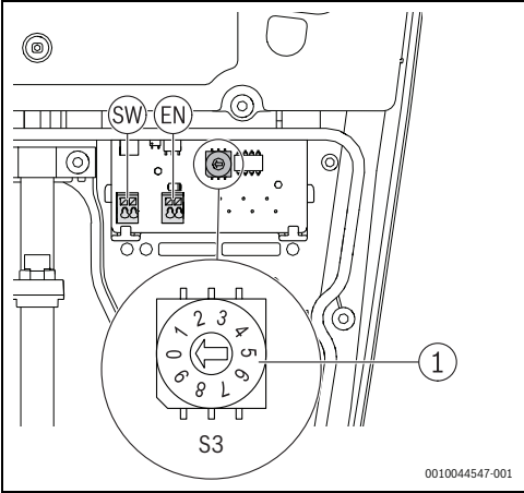
Fig. 110 Selettore di corrente massima (S3)
