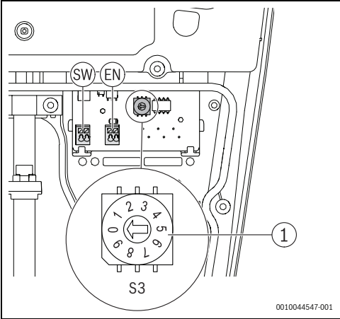
Afb. 134 Keuzetoets max. stroom (S3)
