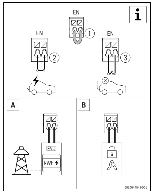
Bild 23 Optionaler Digitaleingang
