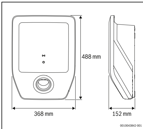
Afb. 124 Productafmetingen
