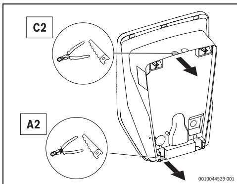
Fig. 178 Capacul racordului electric
