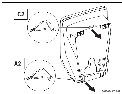
Fig. 82 Capuchon des raccordements électriques
