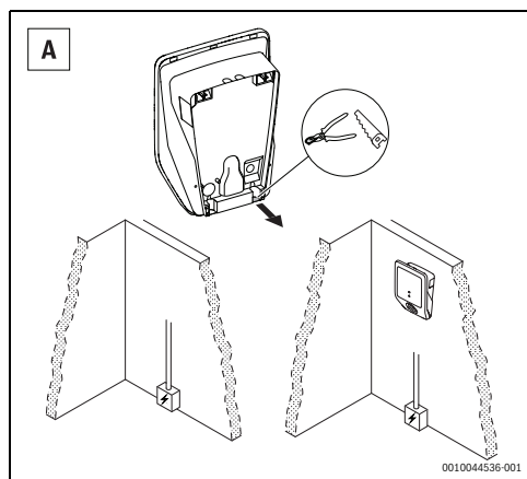
Rys. 150 Przewody zasilania od dołu
