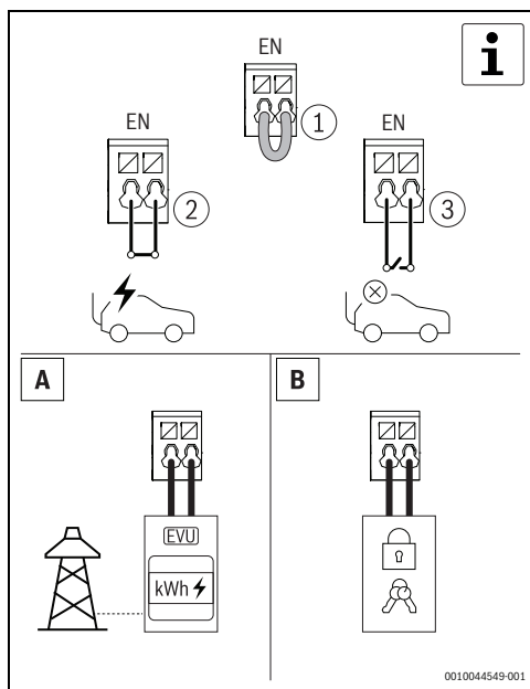
Rys. 167 Opcjonalne wejście cyfrowe
