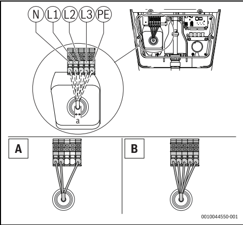
Fig. 85 Alimentation des raccordements électriques A = installation en monophasé B = installation en triphasé
