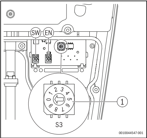
Fig. 86 Bouton de sélection du courant max. (S3)
