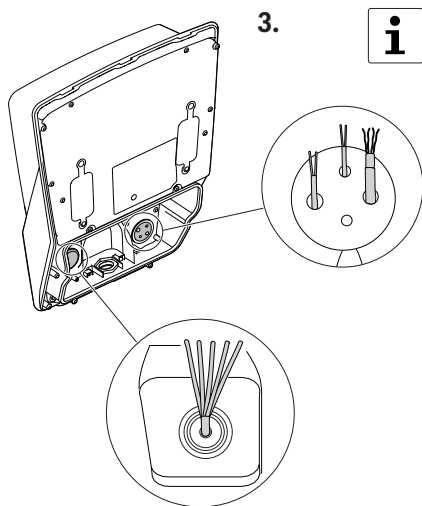
Fig. 84 Montage mural
