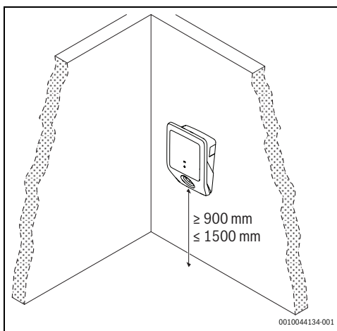
Afb. 125 Minimumafstanden
