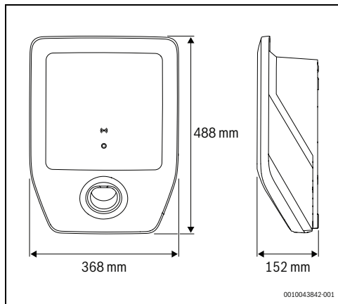
Rys. 148 Wymiary produktu
