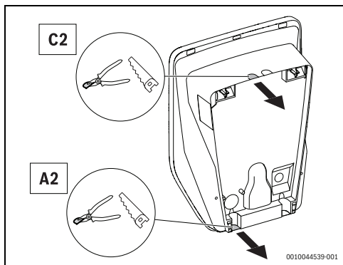
Fig. 106 Tappo dei collegamenti elettrici
