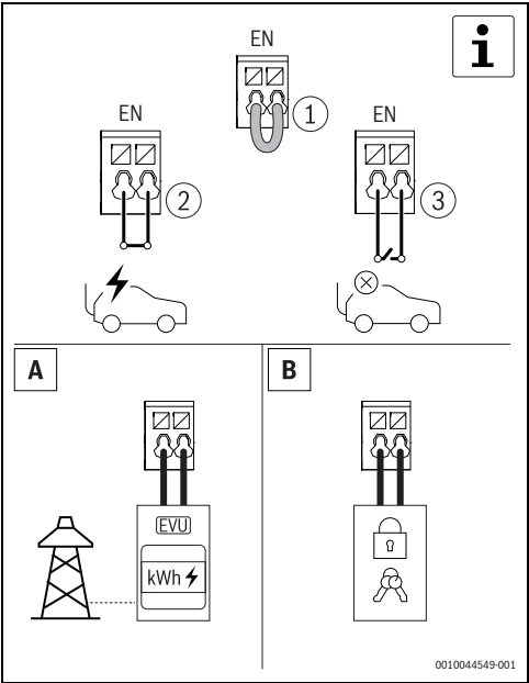
Fig. 95 Entrée numérique en option
