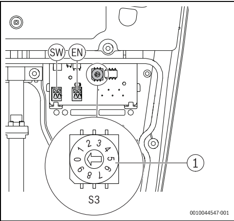
Fig. 182 Buton de selectare al curentului maxim (S3)
