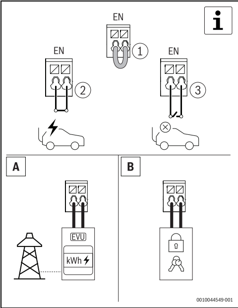
Obr. 215 Voliteľný digitálny vstup
