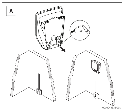
Obr. 30 Napájecí vedení zespodu
