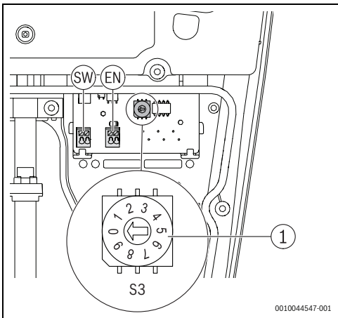
Obr. 38 Přepínač max. proudu (S3)
