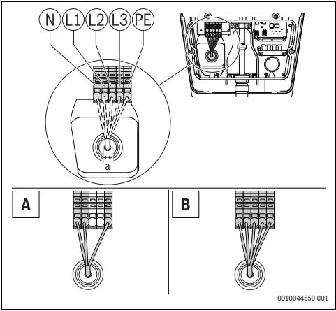
Fig. 109 Collegamenti elettrici alimentazione A = installazione monofase B = installazione trifase
