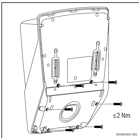
Obr. 209 Inštalácia parkovacieho držiaka
