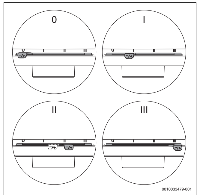
Bild 8 Verbrennungsluftschieber regulieren
