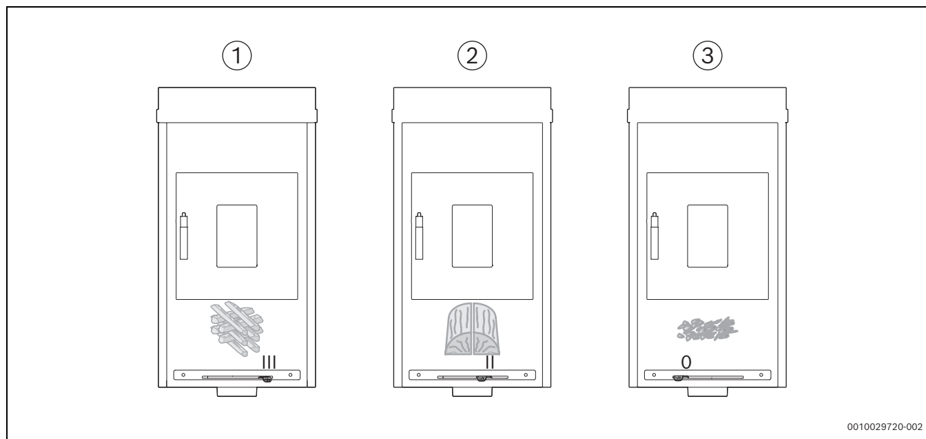
Bild 9 Verbrennungsluftschieber-Stellungen
