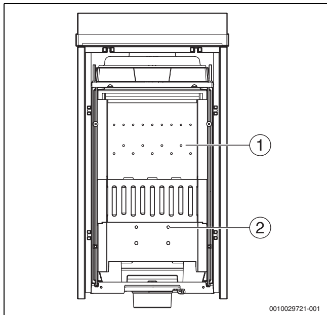
Bild 10 Luftöffnungen
