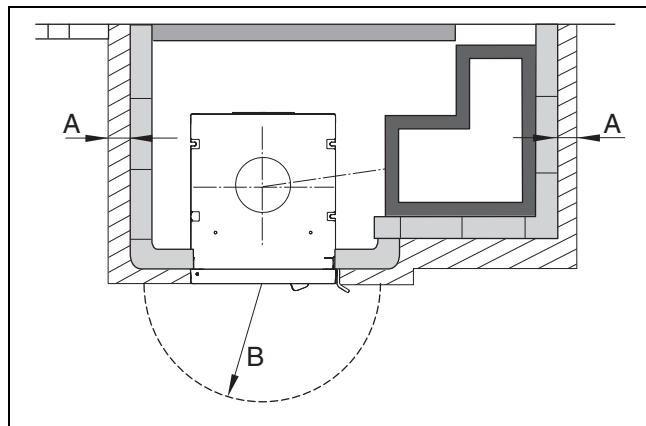
Bild 5 Äußere Mindestabstände
