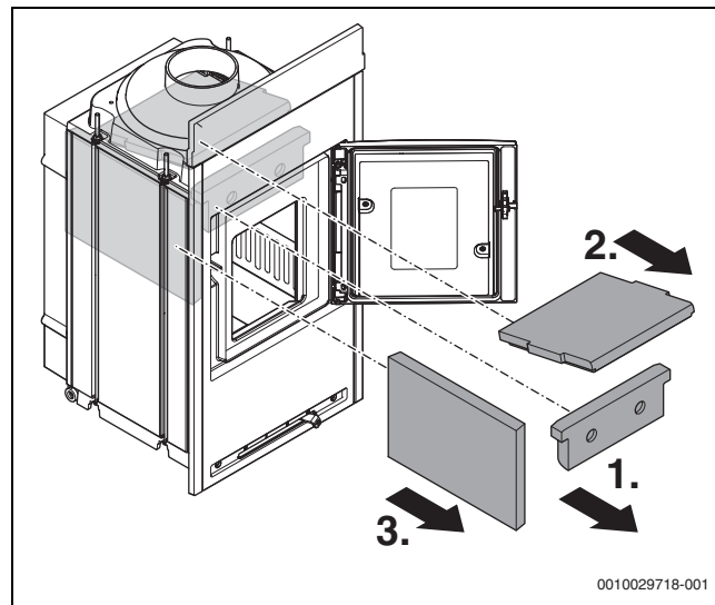
Bild 11 Feuerraumauskleidung ausbauen
