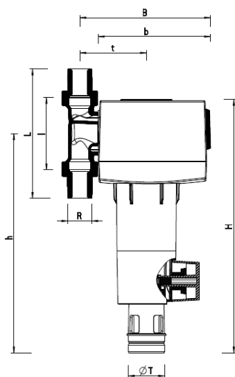
Bild 3: Baumaße Logafix Wasserfilter mit Anschlussstück
