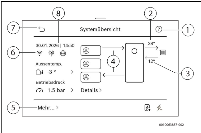
Bild 12 Systemübersicht
