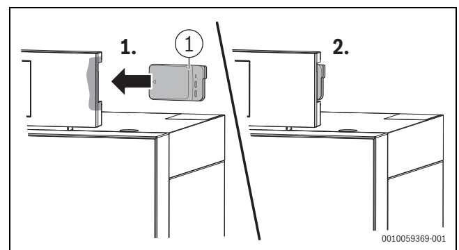
Bild 3 Kommunikationsmodul montieren
