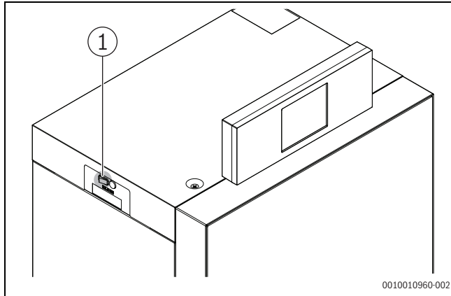
Bild 5 Ein-/Ausschalten
