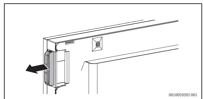
Bild 4 Kommunikationsmodul demontieren
