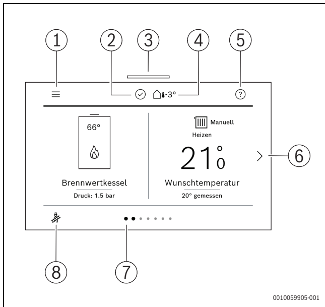
Bild 6 Bedienfeld
