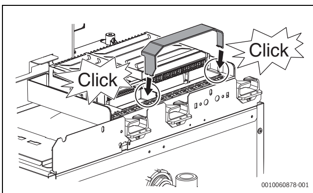
Bild 33 Schutzabdeckung der Anschlüsse aufstecken
