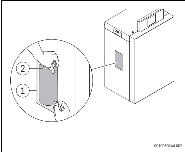
Bild 42 Typschild aktualisieren
