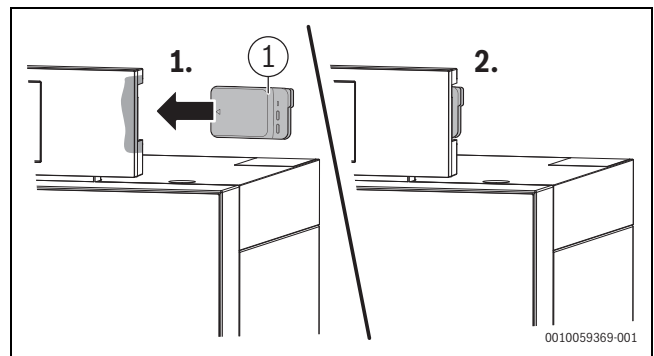
Bild 39 Kommunikationsmodul montieren
