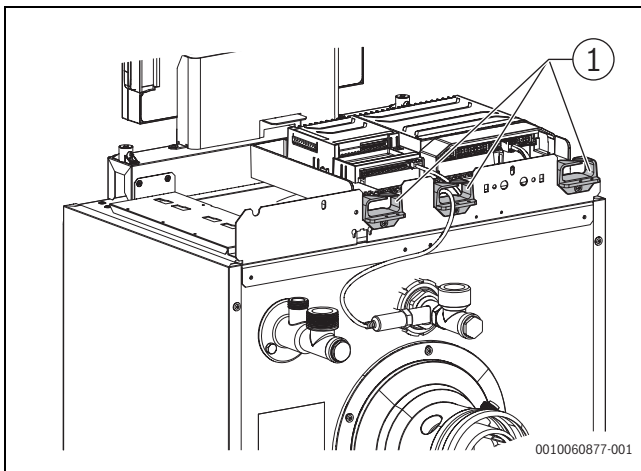
Bild 31 Kabel verlegen
