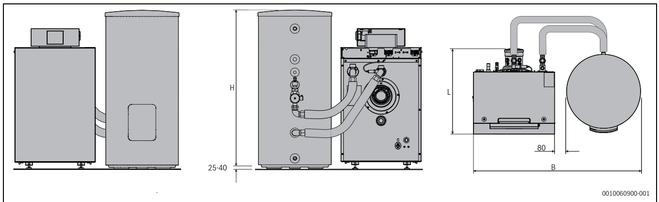
Bild 4 Abmessungen und Anschlüsse Logano plus KBH192i-15...30 mit Logalux SH (Maße in mm)
