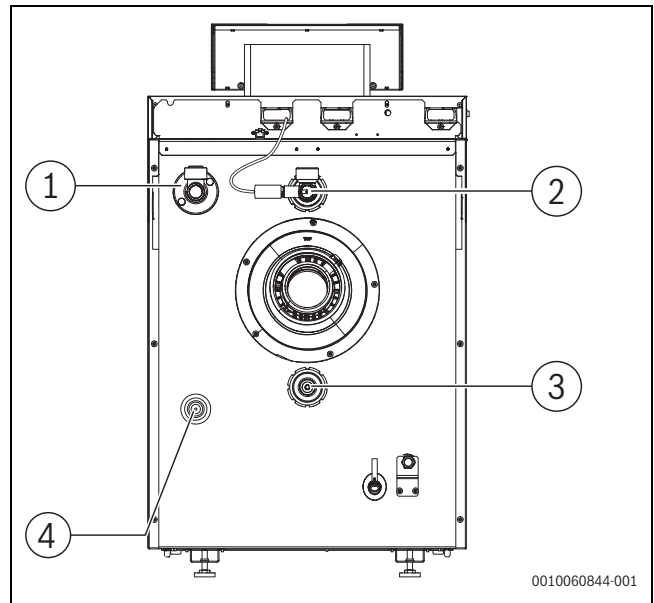
Bild 26 Vorlauf (VK) und Rücklauf (RK) montieren
