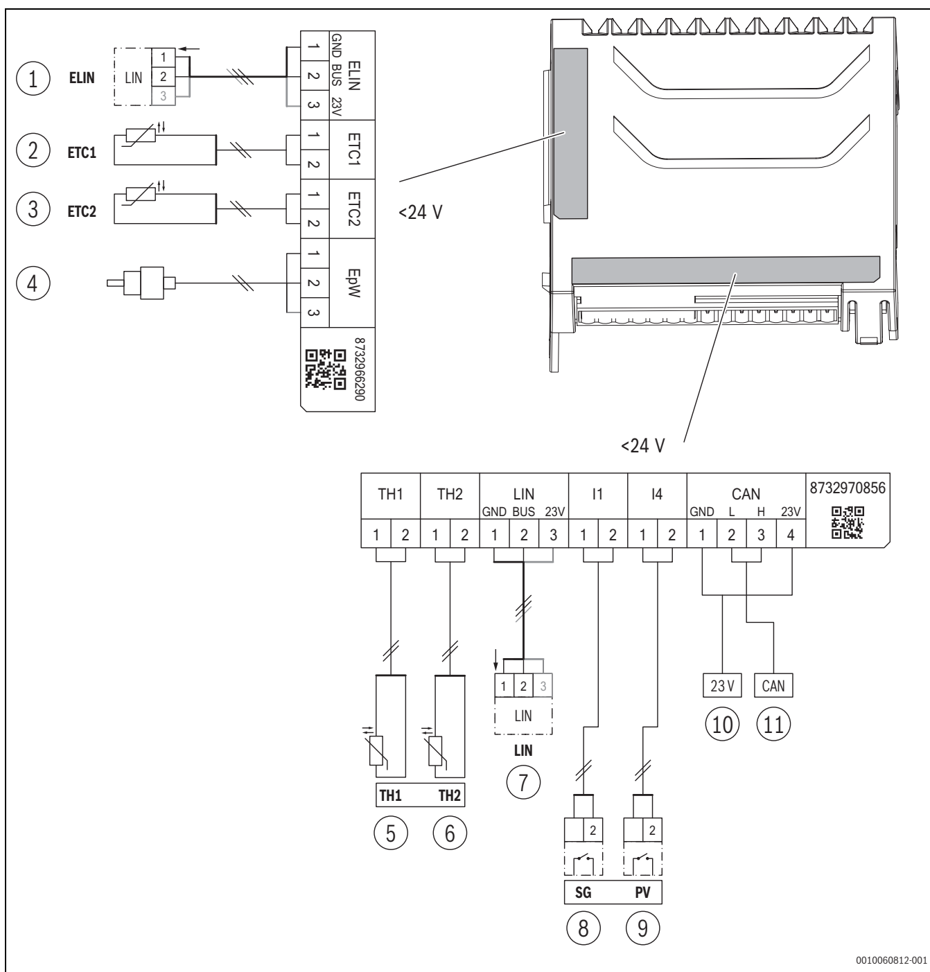
Bild 82 Anschlussplan Hybridmodul IMH200
