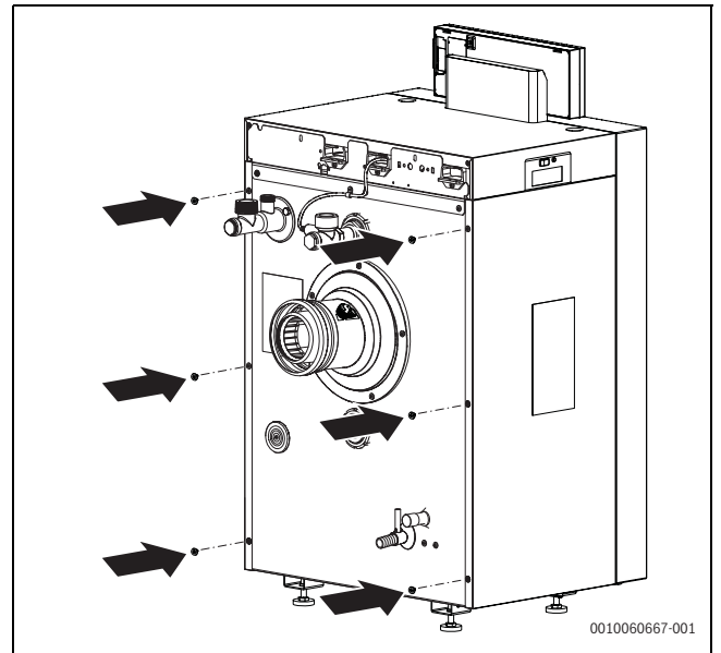
Bild 14 Seitenwände befestigen
