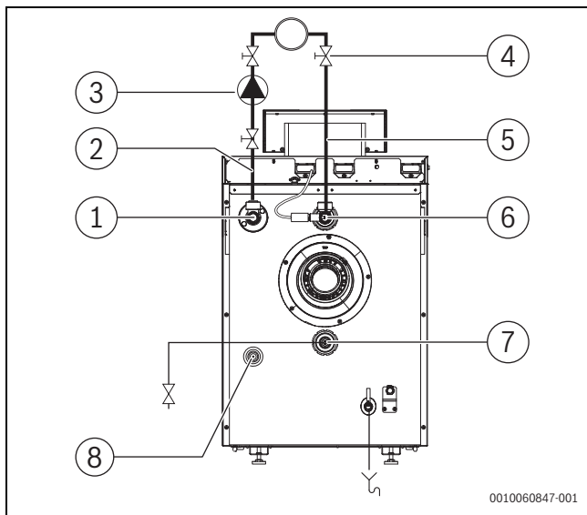
Bild 25 Anschlusschema Hydraulik
