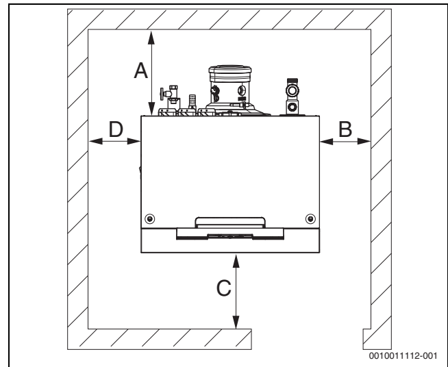
Bild 16 Wandabstände im Aufstellraum
