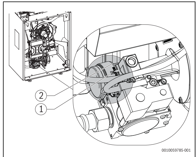
Bild 43 Einstelldüse Gasarmatur
