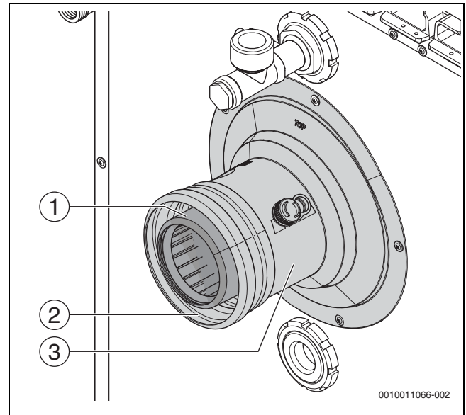
Bild 21 Abgasanschluss montieren
