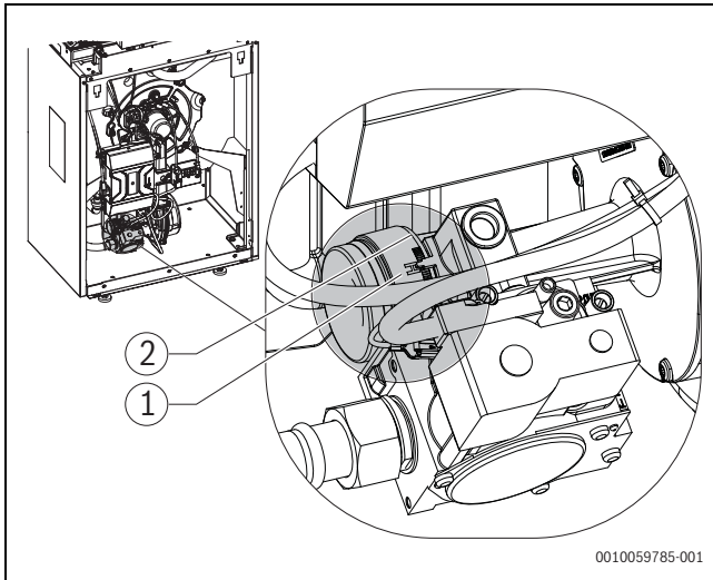
Bild 48 Einstelldüse Gasarmatur
