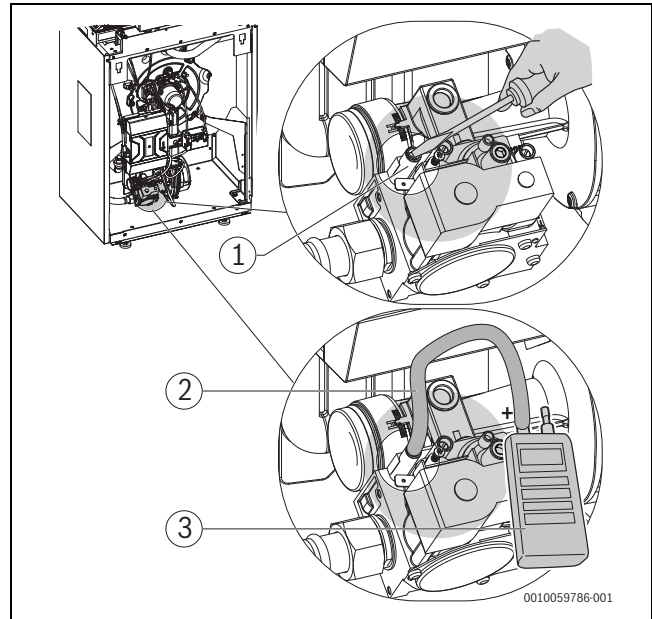
Bild 55 Gas-Anschlussdruck messen
