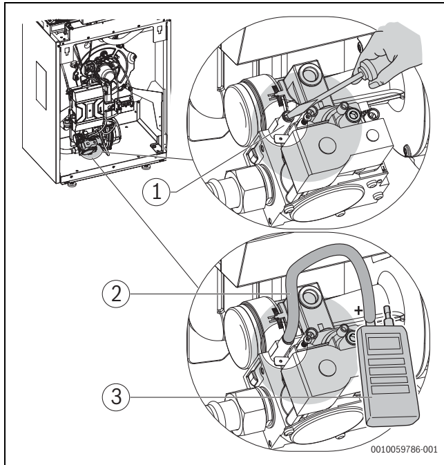
Bild 47 Gas-Anschlussdruck messen
