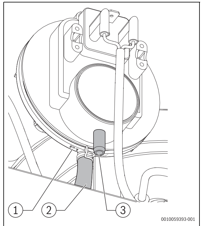
Bild 74 Detailansicht ADS-Druckschalter
