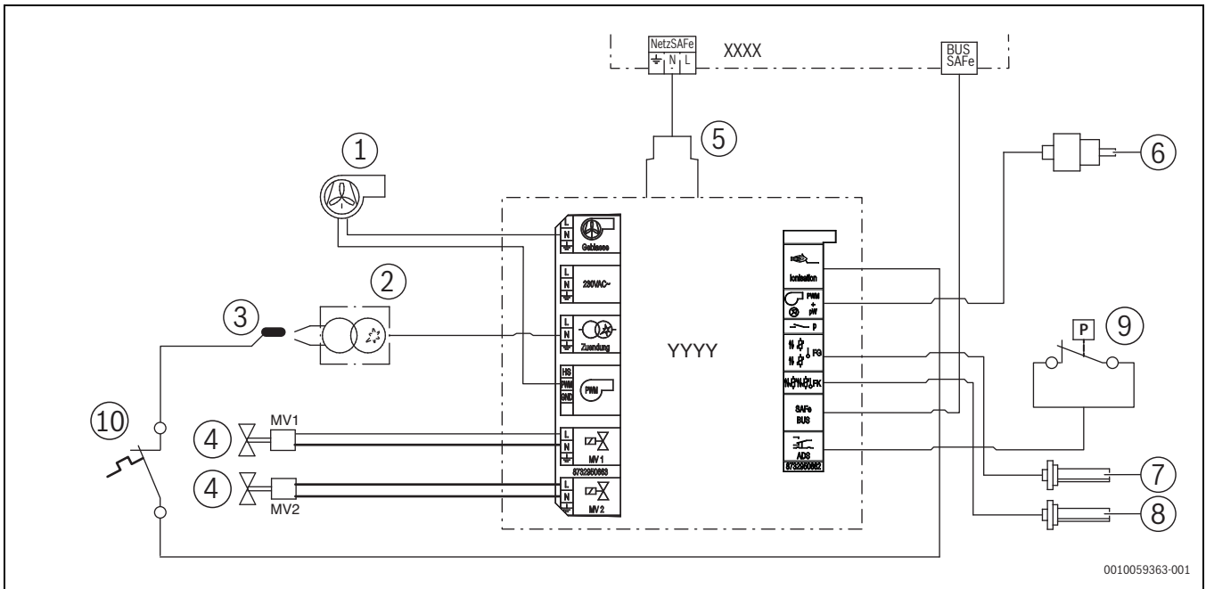
Bild 85 Anschlussplan Feuerungsautomat
