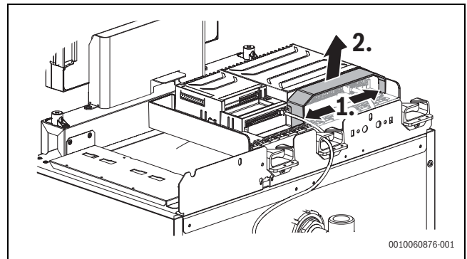
Bild 30 Schutzabdeckung der Anschlüsse abnehmen
