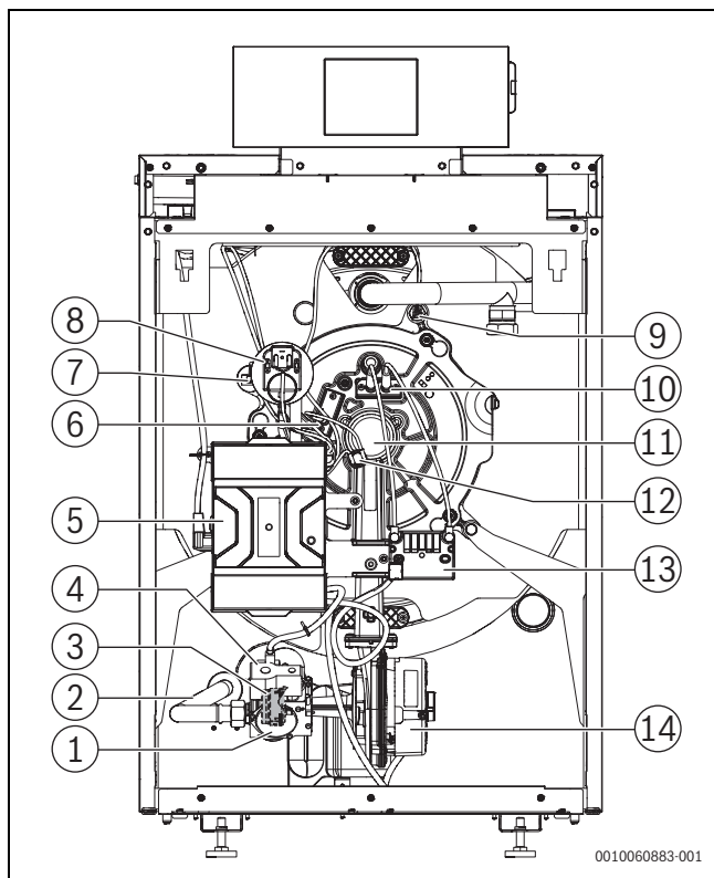
Bild 79 Vorderansicht
