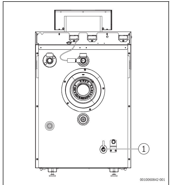
Bild 24 Kondensatschlauch montieren
