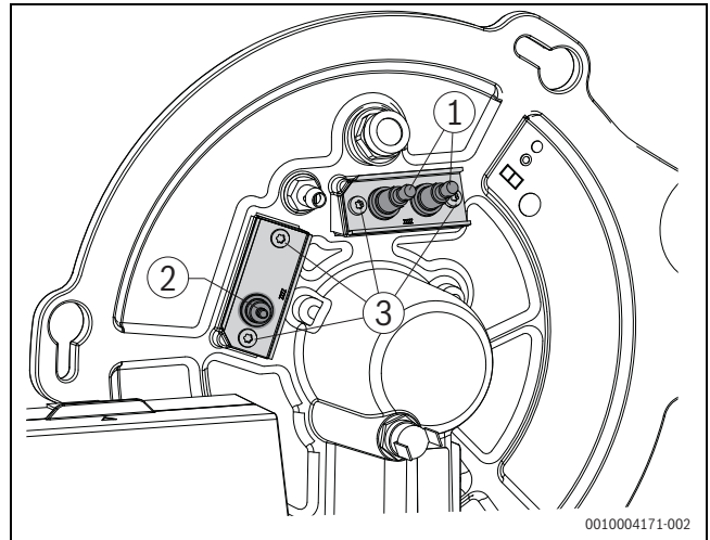
Bild 67 Elektrodenposition
