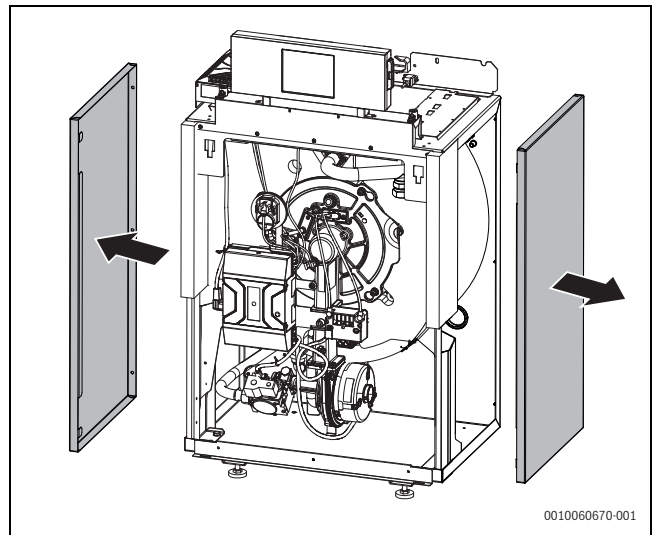
Bild 11 Seitenwände abnehmen
