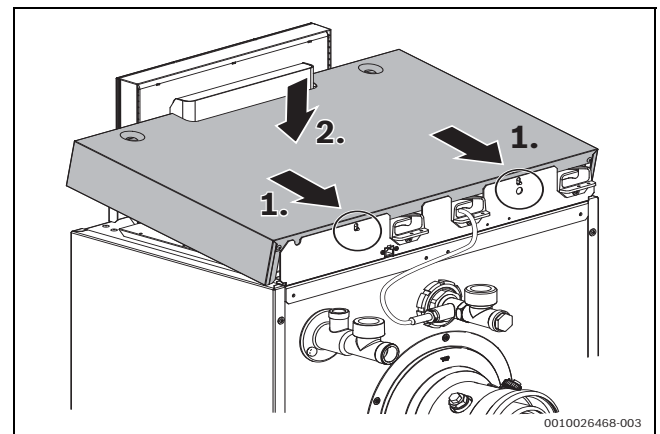
Bild 34 Kesselhaube montieren
