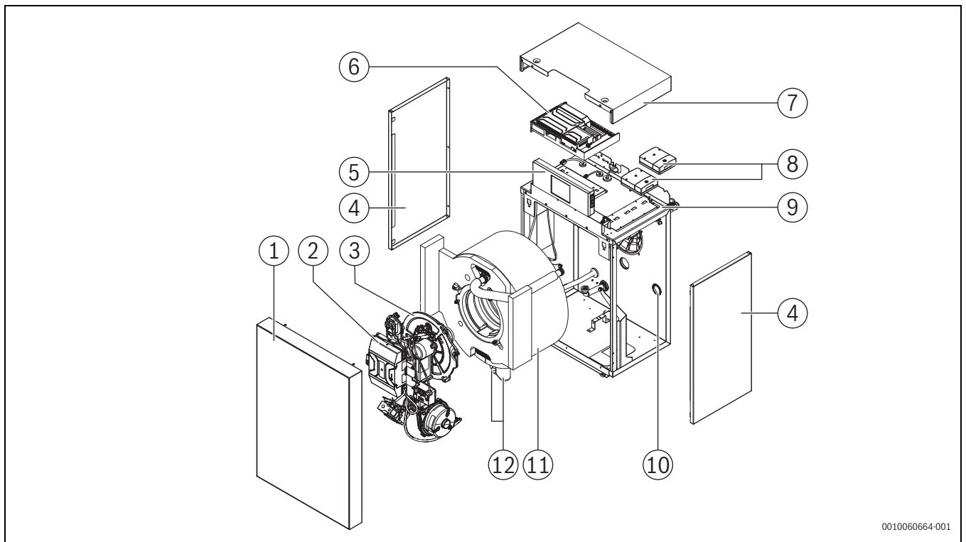
Bild 1 Logano plus KBH192i-15...30 – Hauptbestandteile
