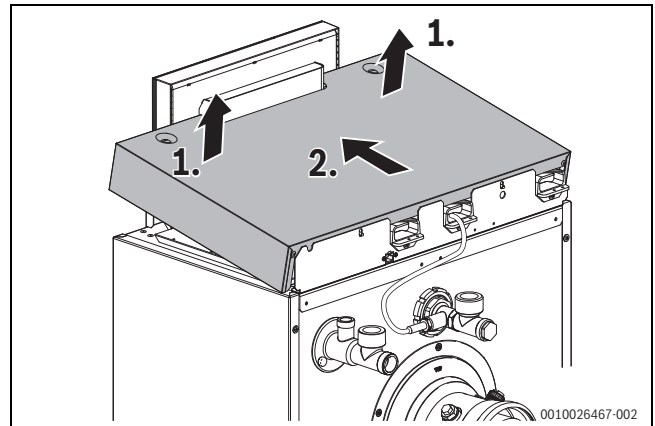
Bild 29 Kesselhaube abnehmen
