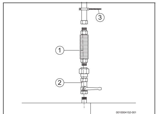
Bild 28 Gasanschluss herstellen
