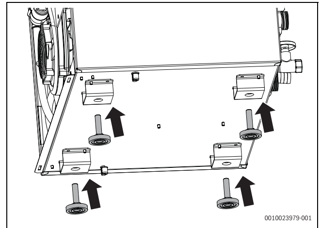
Bild 18 Stellfüße montieren
