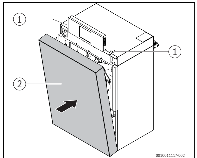
Bild 15 Kesselvorderwand montieren
