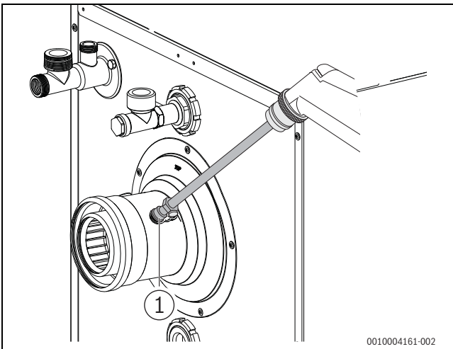
Bild 53 Messwerte aufnehmen
