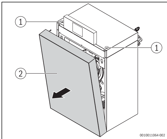
Bild 17 Kesselvorderwand demontieren
