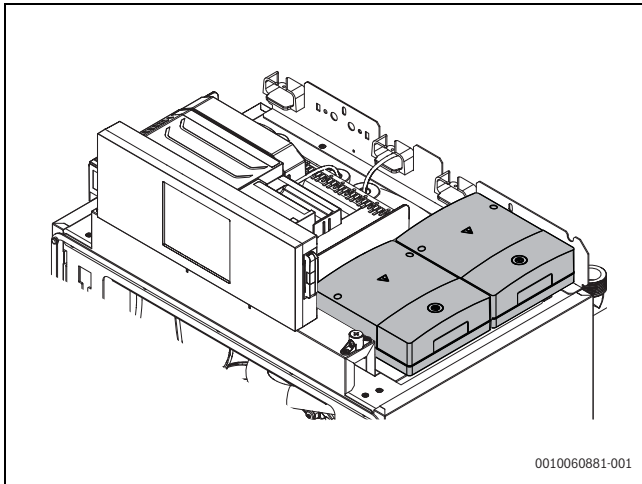
Bild 37 Standard-Funktionsmodule montiert
