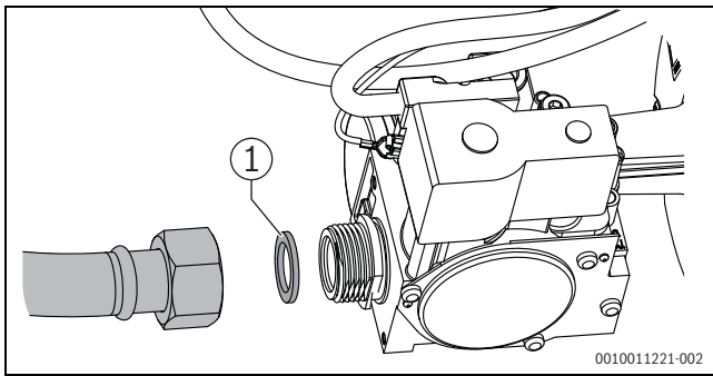
Bild 61 Gasrohr abnehmen
