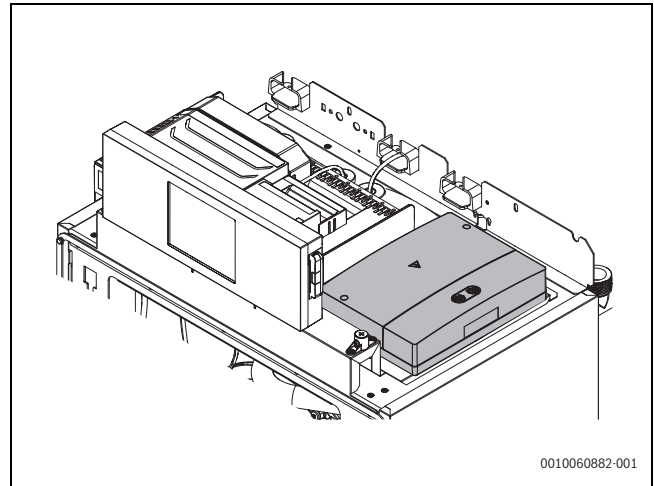
Bild 38 Großes Funktionsmodul montiert
