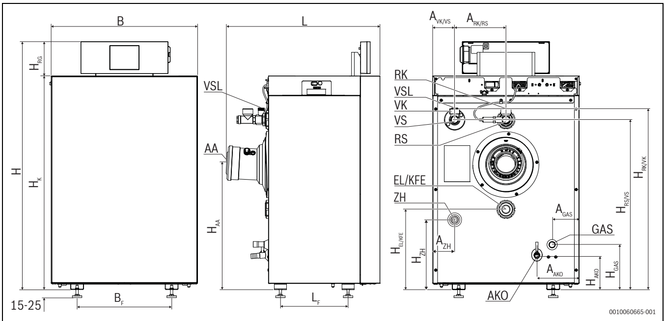
Bild 3 Abmessungen und Anschlüsse für Logano plus KBH192i-15...30 (Maße in mm)
