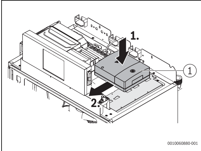
Bild 36 Funktionsmodule einstecken
