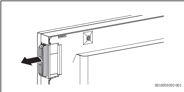
Bild 40 Kommunikationsmodul demontieren
