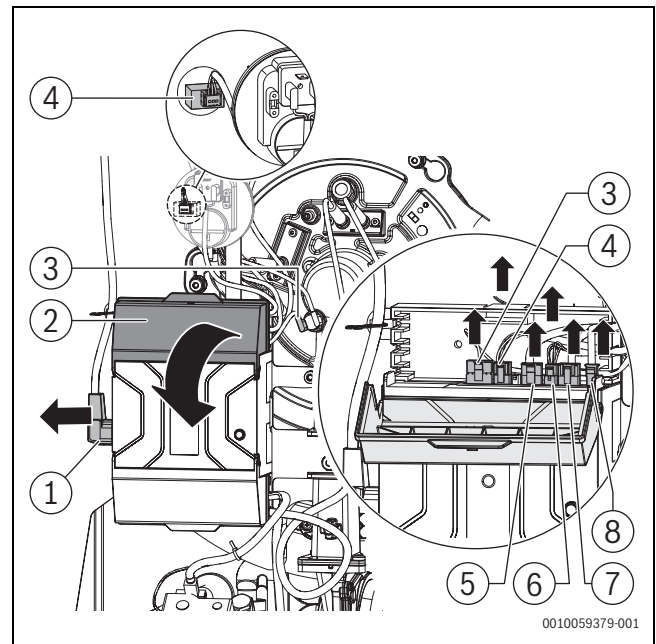
Bild 59 Steckverbinder lösen
