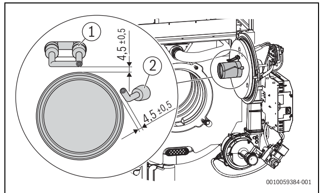
Bild 68 Abstände Elektroden
