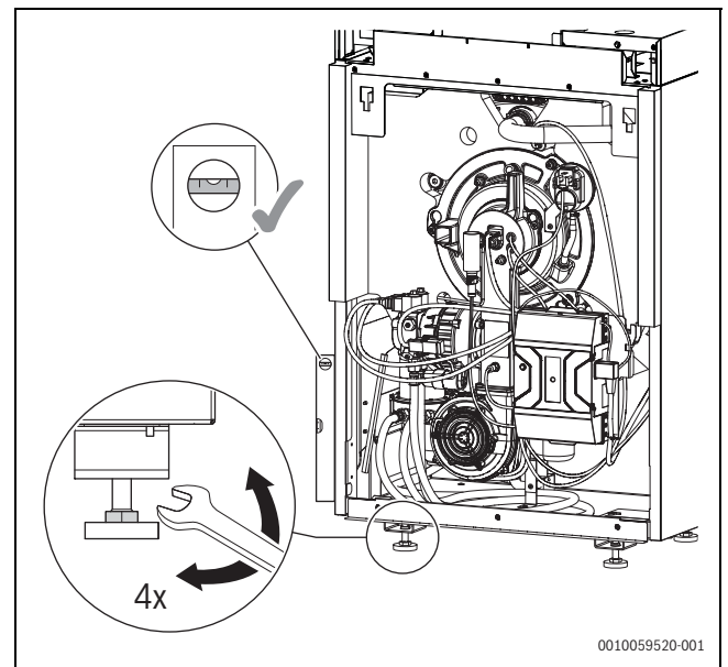
Bild 19 Heizkessel ausrichten
