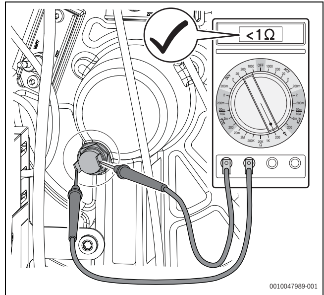
Bild 77 Elektrischen Widerstand an den Kontakten des Temperaturwächters messen (Temperaturwächter in Ordnung)
