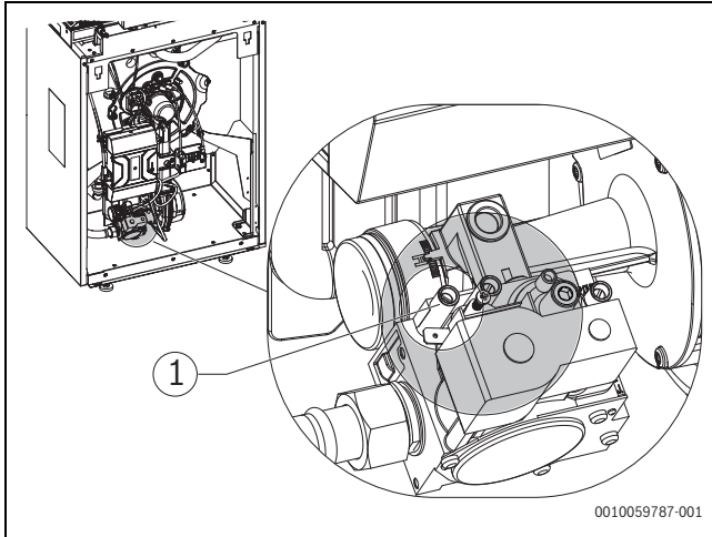
Bild 44 Gasleitung entlüften
