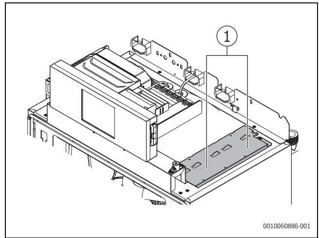
Bild 84 Ansicht ohne Abdeckhaube und ohne Module
