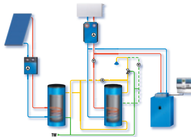
Anlagenbeispiel 2: Zweispeicheranlage mit Vorwärmstufe für die solare Trinkwassererwärmung
