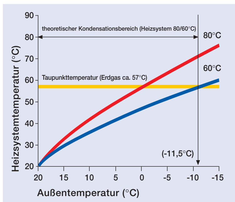
Bild 2: Gas-Brennwertnutzen bei Heizsystem 80/60^\circ\text{C}
