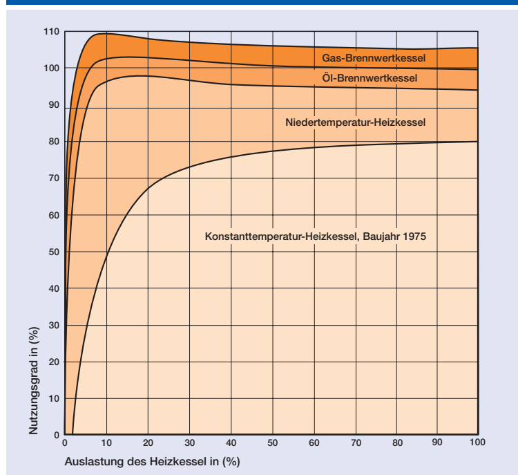
Bild 1: Teillast-Nutzungsgradverläufe von Heizkesseln
