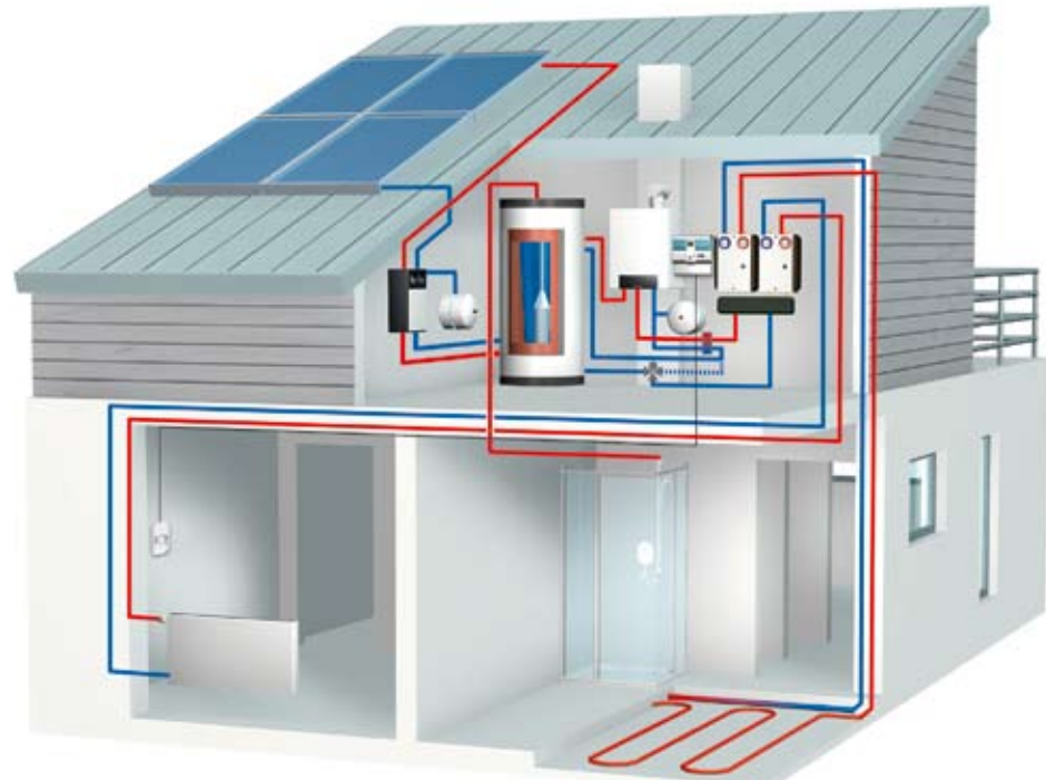
Bild 1 Bei intelligenter Einbindung der solaren Heizungsunterstützung ist die Gesamtanlage viel mehr als die Summe ihrer Einzelkomponenten
