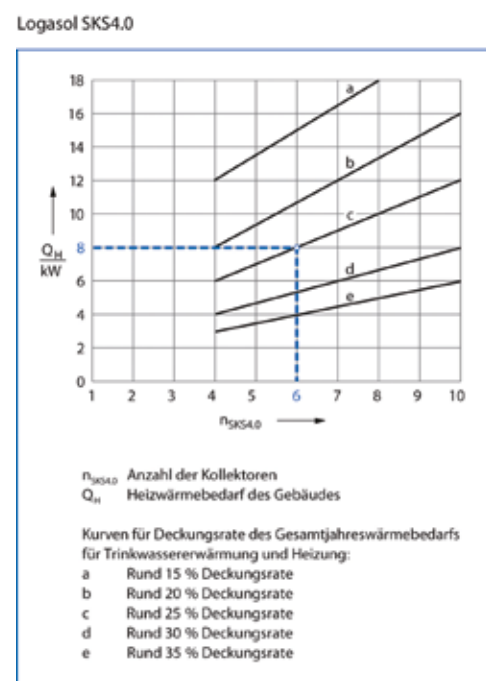
Bild 2 Überschlägige Bestimmung der Kollektoranzahl einer Solaranlage mit Heizungsunterstützung in Abhängigkeit der gewünschten solaren Deckungsrate und der maximalen Gebäudeheizlast
