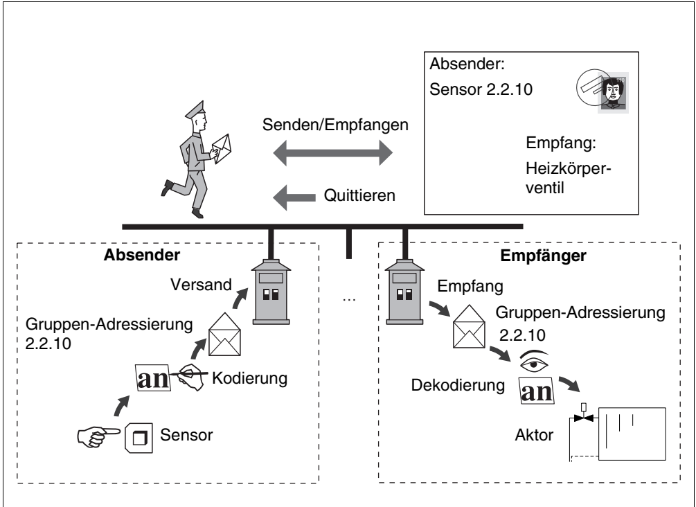
Abb. 1 Datenübertragung – Beispiel
