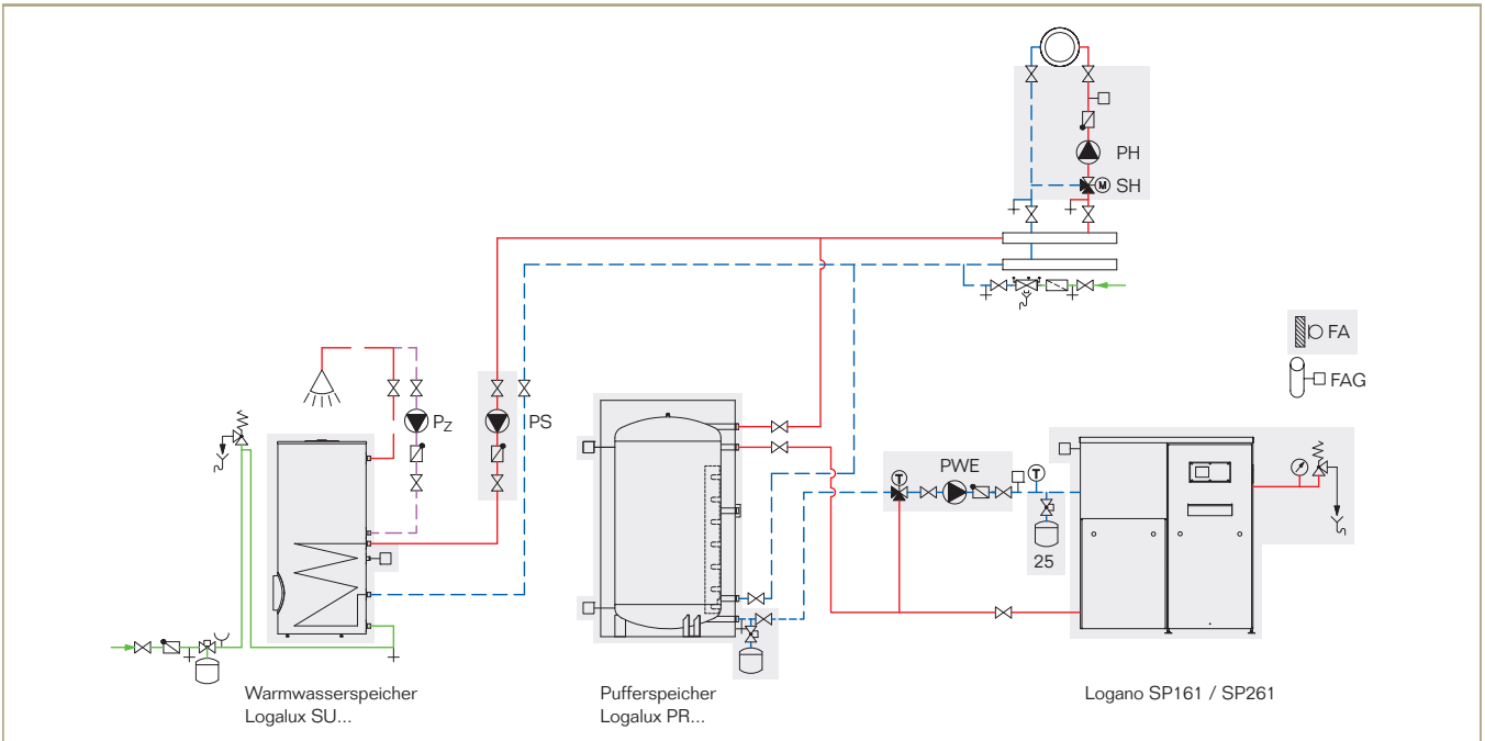
Hydraulik Beispiel mit Pufferspeicher und Warmwasserbereitung
