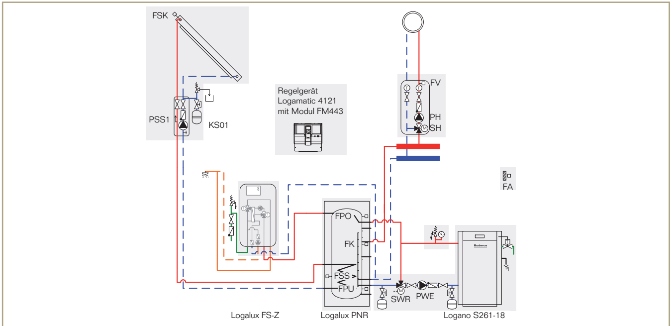
Hydraulik Beispiel mit Pufferspeicher und Warmwasserbereitung
